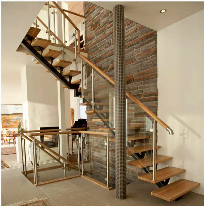
Räcke Glas 8 mm. Räckesstolpar i borstat rostfritt stål, profil rund 40 mm i diameter. Handledare (överliggare) i trä, profil rund. Avslut handledare hylsa rak/välvd i borstat rostfritt stål.
