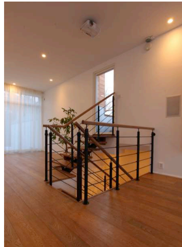
Räcke Marin. Utförande i pulverlackat stål, RAL kulörschema. Antal medlöpare 8 mm, 5 styck. Handledare fyrkantsprofil med översida välvd.
