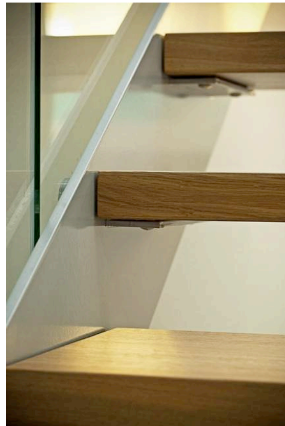
Kontor. L-formad trappa modell Nordic Light inklusive vilplan. Sidovangstycken i pulverlackat stål RAL kulörschema. Steg i semi matt lackad ek. Räcke i trappa samt runt bjälklagsöppning glasträcke 13 mm – härdat och laminerat. Handedare räcke fyrkantsprofil 50 x 50 mm.
