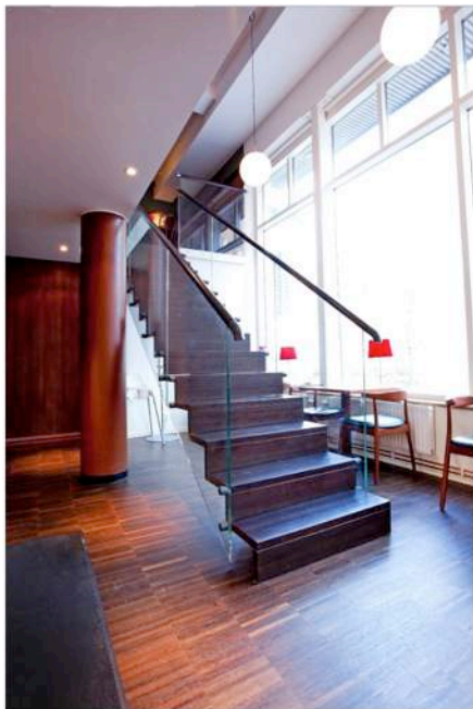
Café. Rak enbalkstrappa med underliggande balk i pulverlackat stål, RAL kulörschema. Profil balk zigzag. Sätt- & plansteg i betsad och semimatt lackad ek. Räcke i trappa samt runt bjälklagsöppning glasträcke 13 mm – härdat och laminerat. Handledare räcke rundstav 50 mm i diameter.
