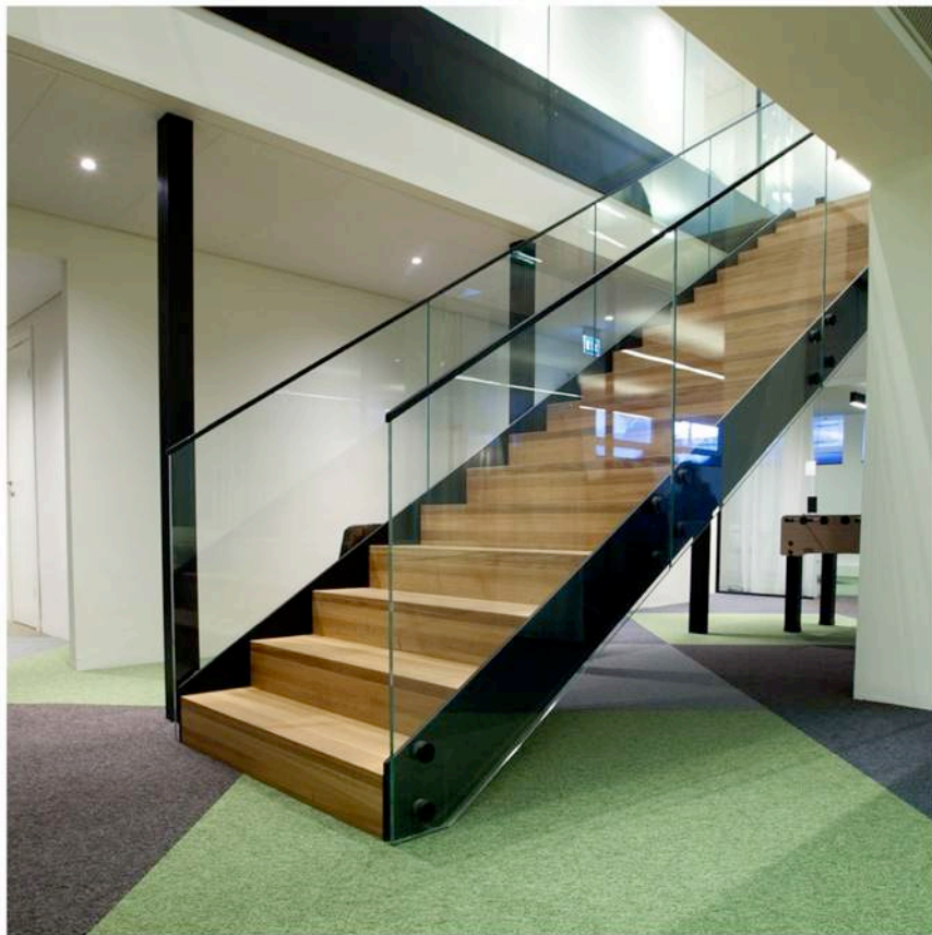
Kontor. Rak frihängande trappa modell Nordic Light, med sidovangstycken i pulverlackat stål RAL kulörschema. Räcke i trappa samt runt Bjälklagsöppning glasträcke 13 mm – härdat och laminerat. Glasets överkant omslutet av stålprofil pulverlackat RAL kulörschema.
