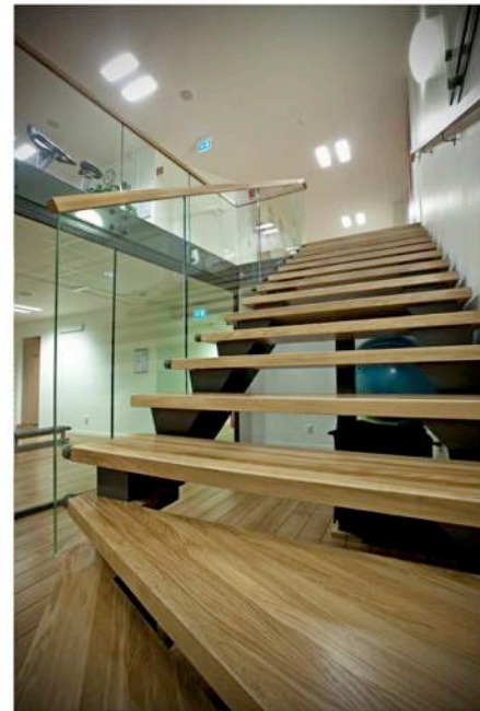
Gym. L-formad tvåbalkstrappa med sidmonterat glasträcke 13 mm – härdat och laminerat. Underliggande balkar profil rak, pulverlackade RAL kulörschema. Steg i semi matt lackad ek. Överliggare (handledare) i 50 mm profil fyrkant, utförande och finish samma som steg.
