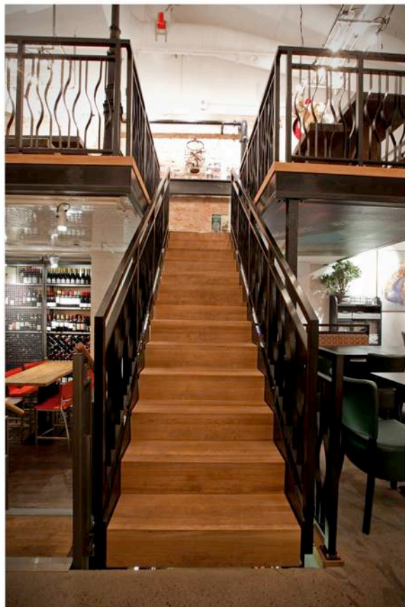
Restaurang. Två trappor – rak respektive L-formad – modell Nordic Light med sidovangstycken i pulverlackat stål RAL kulörschema. Sätt- & plansteg i semi matt lackad ek. Räcke och handledare modell smide pulverlackade RAL kulörschema.
