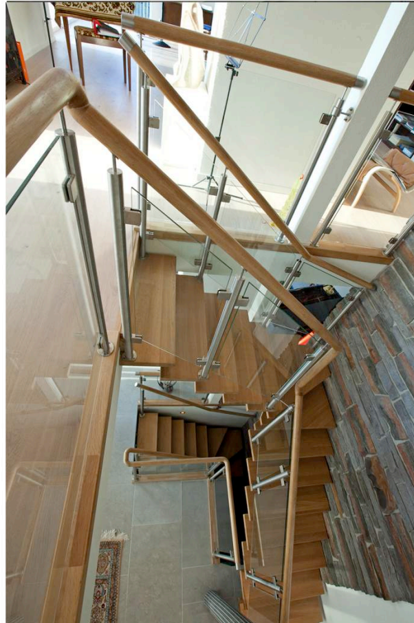
L-formad enbalkstrappa med räcke Glas 4 + 4 mm laminerat. Steg i semi matt lackad ek. Underliggande balk rak profil, pulverlackad kulör RAL kulörschema. Handledare räcke diameter 50 mm.
