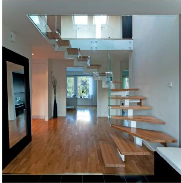
U-formad enbalkstrappa med räcke Glas 13 mm härdat och laminerat. Steg i semi matt lackad ek. Underliggande balk zigzag profil, pulverlackad kulör RAL kulörschema.
